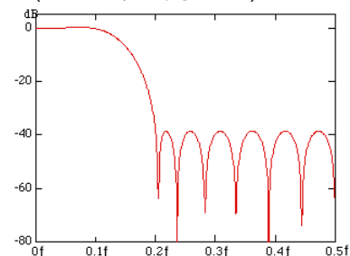
FIR(Low Pass, カットオフ10%)
