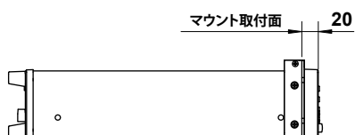
●EIA ラックマウント取付寸法
