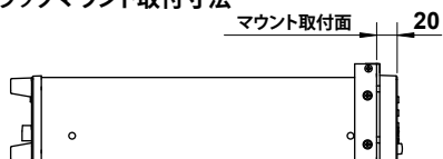
●JIS ラックマウント取付寸法
