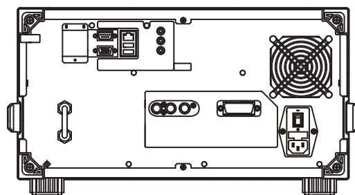
背面図
