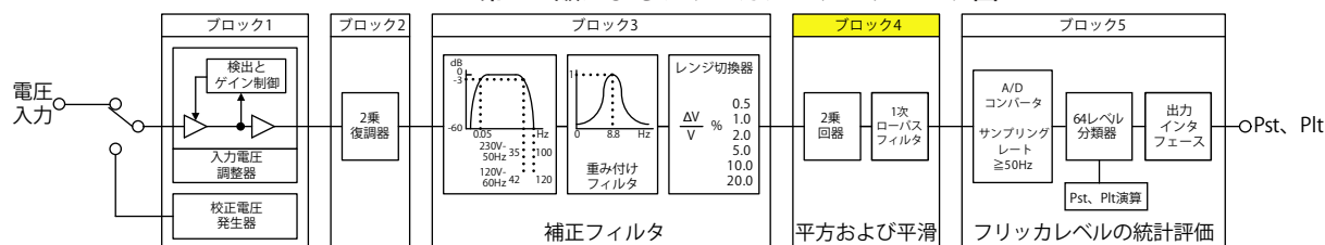
IEC 61000-4-15 第 1.1 版によるフリッカメータのブロック図
