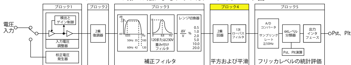
IEC 61000-4-15 第 2.0 版によるフリッカメータのブロック図
