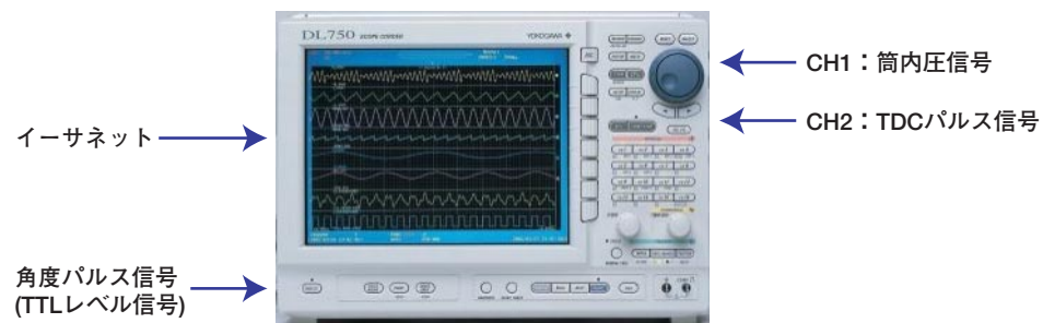
信号接続図
