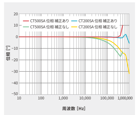
位相特性例
