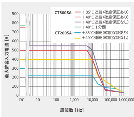
ディレーティング特性例
