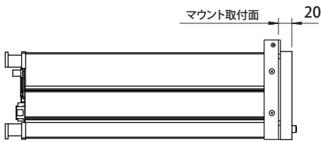
JIS ラックマウント取付寸法
