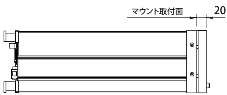
EIA ラックマウント取付寸法
