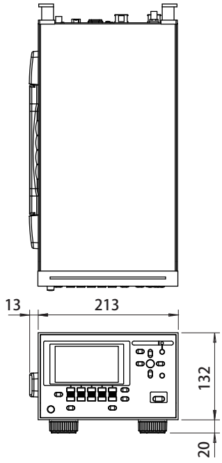
JIS ラックマウント取付寸法
