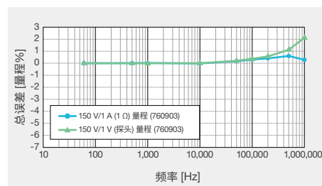
零功率因数下的频率—功率精度特性
