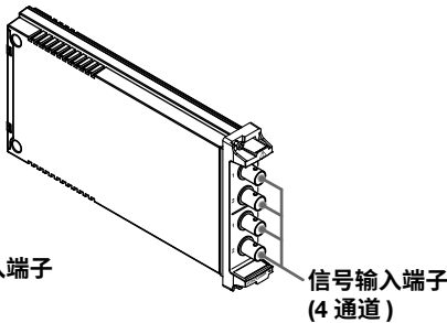
通用 (电压 / 温度) 模块 UNIVERSAL (型号 : 701261)
