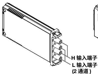
高电压 1MS/s 16-Bit 绝缘模块 (带 AAF 和 RMS) HV (AAF、RMS) (型号 : 720268)
