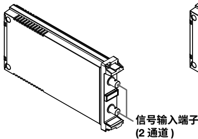
高速 100MS/s, 12-Bit 绝缘模块 HS100M12 (型号 : 720211)
