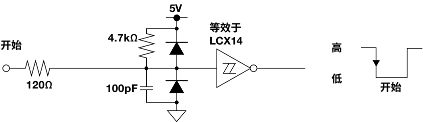
信号输入电路
