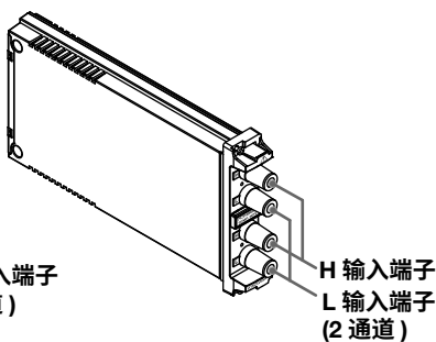
通用 (电压 / 温度) 模块 UNIVERSAL (型号 : 701261)
