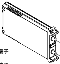
SENT 监视模块 SENT (型号 : 720243)
