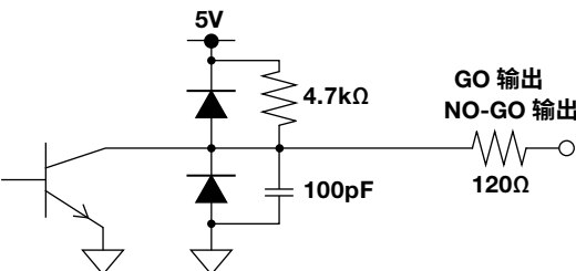
信号输出电路
