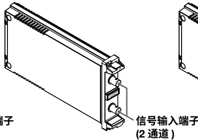
高速 10MS/s, 12-Bit 绝缘模块 HS10M12 (型号 : 720250)
