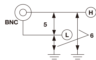
直接输入 (不符合安全标准的电缆)
