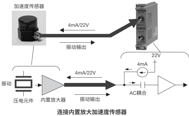
连接内置放大加速度传感器
