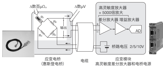
应变片和测量电路
