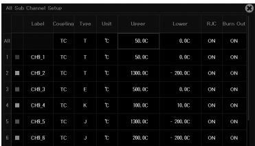
通道设置画面（DL950）
