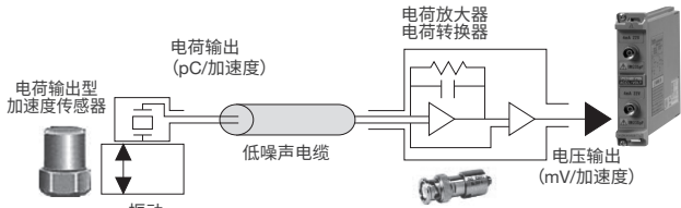
连接电荷输出型加速度传感器
