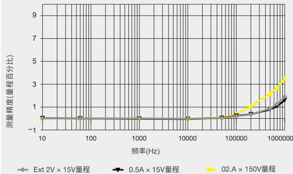
测量精度(量程百分比) vs 频率(Hz)(功率因数=0)
