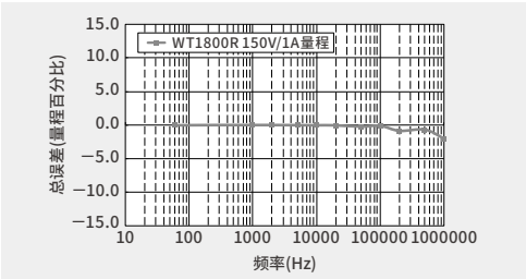
功率因数为零时的频率-功率精度特性示例
