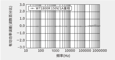
功率因数为1时的频率-功率精度特性示例
