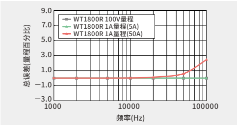
共模电压对读数的影响示例
