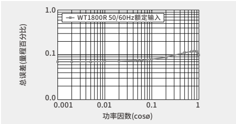
任意功率因数下额定量程输入的总功率误差(50/60Hz时)
