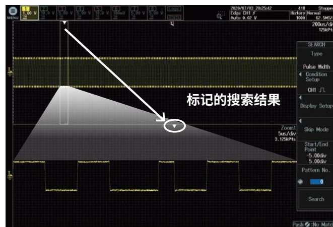
按脉宽搜索波形
